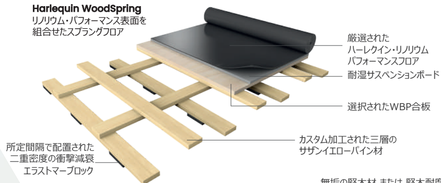
Harlequin WoodSpring 堅木張りまたはエンジニアボード 張りのスプリングフロア
