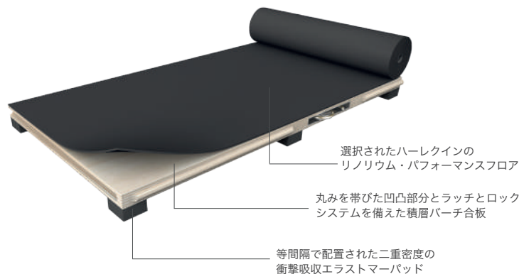
ハーレクイン独自のラッチとロックシステム
