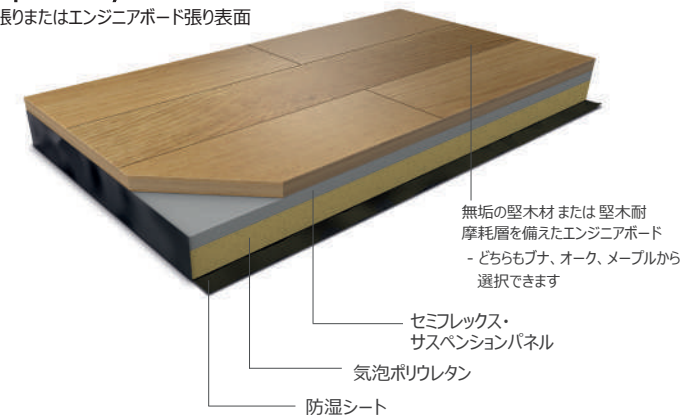
Harlequin Activity スプリングフロア 堅木張りまたはエンジニアボード張り表面
